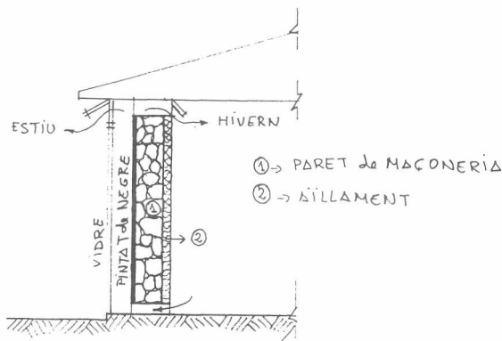
EXEMPLE DE PARET COL·LECTORA
