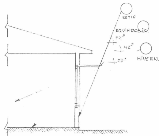
EXEMPLE DE VOLADÍS
