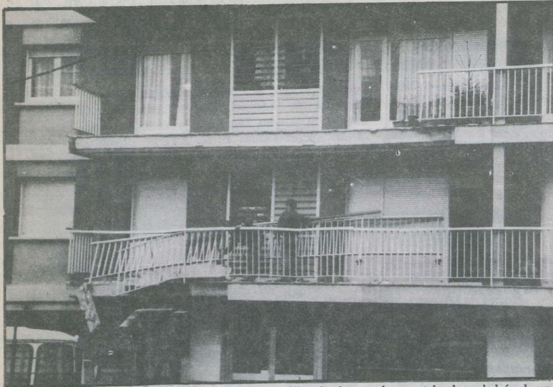
Tal como puede apreciarse en la fotografía, la barandilla y la obra que la soportaba de un balcón de un segundo piso cayó sobre el primero, y posteriormente sobre un vehículo aparcado en la calle, produciendo daños de considerable valor. El accidente ocurrió en un edificio de reciente construcción, al final del carrer nou, en la plaza de la Creu de la Mà, a mediodía del martes de la semana pasada. No se registraron desgracias personales.
