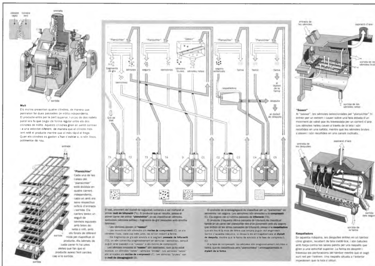
Dibuix d'un molí a cilindres o triturador. Quaderns de Didàctica i Difusió del Museu de la Ciència i de la Tècnica de Catalunya.
