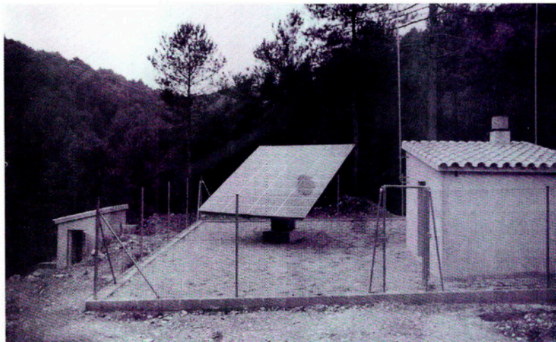
La planta de captació d'energia solar fotovoltaica per al bombeig municipal d'aigua, tot i que no fou una solució definitiva, va suposar una experiència pilot a l'Estat.
