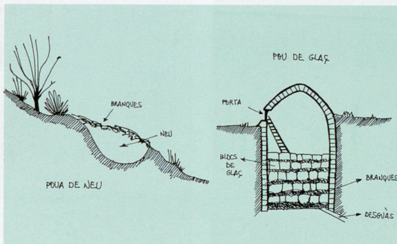
Dibuix esquemàtic d'un pou de glaç i d'una poua de neu o congesta.
