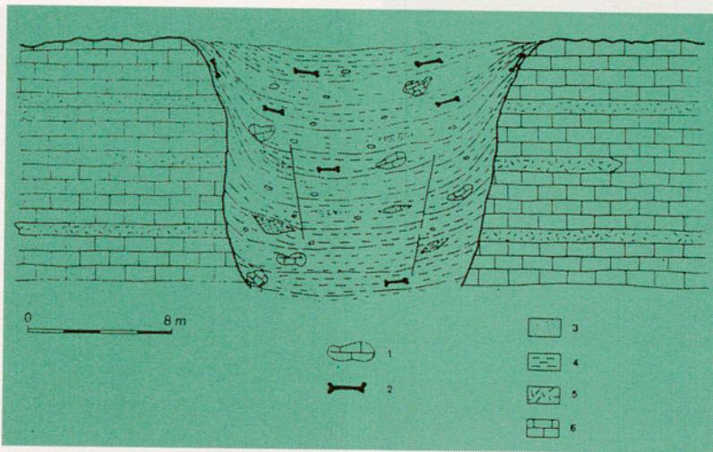
Secció esquematitzada d'un farcit dels embuts (adaptat de Julià & Villalta, 1984. 1: Fragments de calcisilitites. 2: Restes d'ossos. 3: sorres. 4: argiles. 5: travertí de caràcces. 6: calcisilitites.
