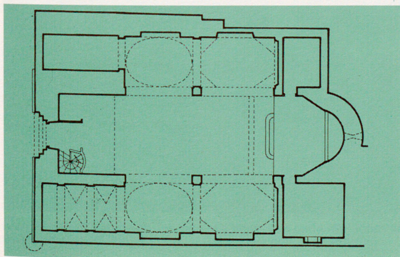
Planta de l'església parroquial.
