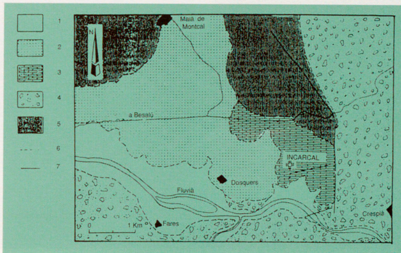
Situació geològica de la regió: 1. Quaternari indiferenciat; 2. Glacis de Maià de Montcal; 3. Calç lacustre d'Incarcal; 4. Pliocè detrític; 5. Eocè; 6. Contacte discordant, i 7. Falla (croquis adaptat de Julià, 1980).
