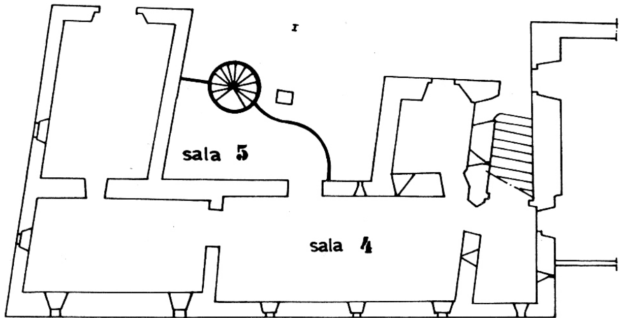
PLANTA BAIXA
