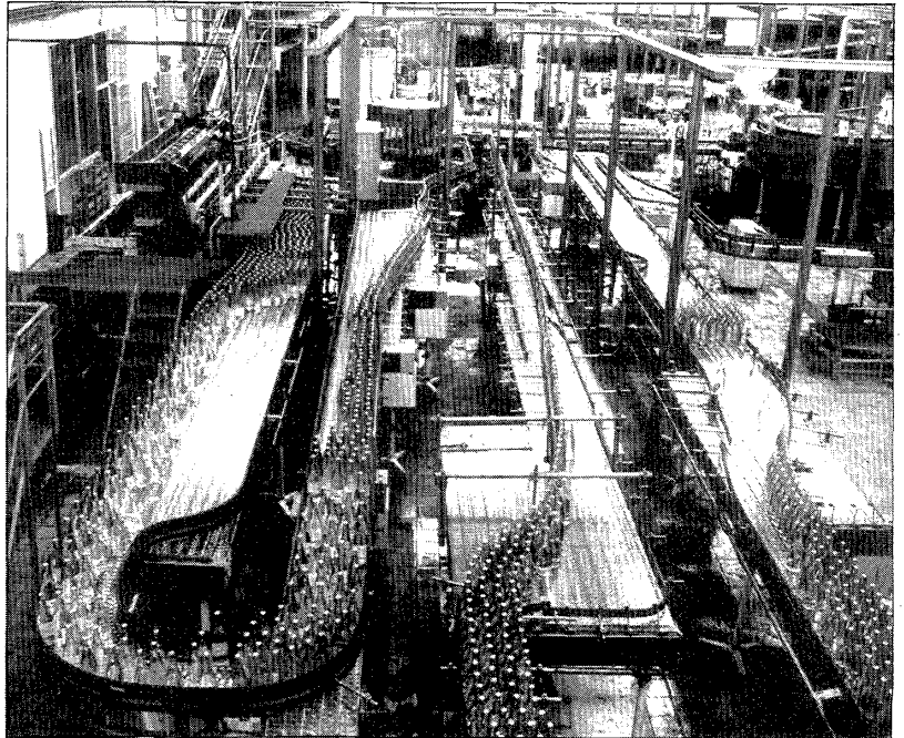
Aspecte interior de la cadena d'una planta d'envasament d'aigües minerals
