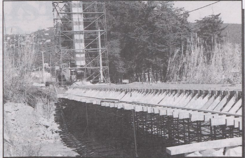
■ Una aspecte del pont projectat per l'enginyer Eduard Folqué en una etapa de la seva construcció.
