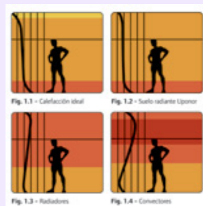
> Corbes de temperatura segons sistema de calefacció (Manual técnico de climatización invisible - Uponor)
